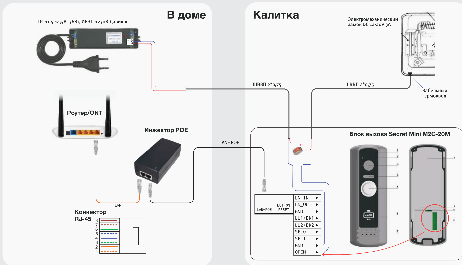
Схема подключения вызывной панели DK8252-Doorbell CCDCAM по UTP с POE-инжектором
